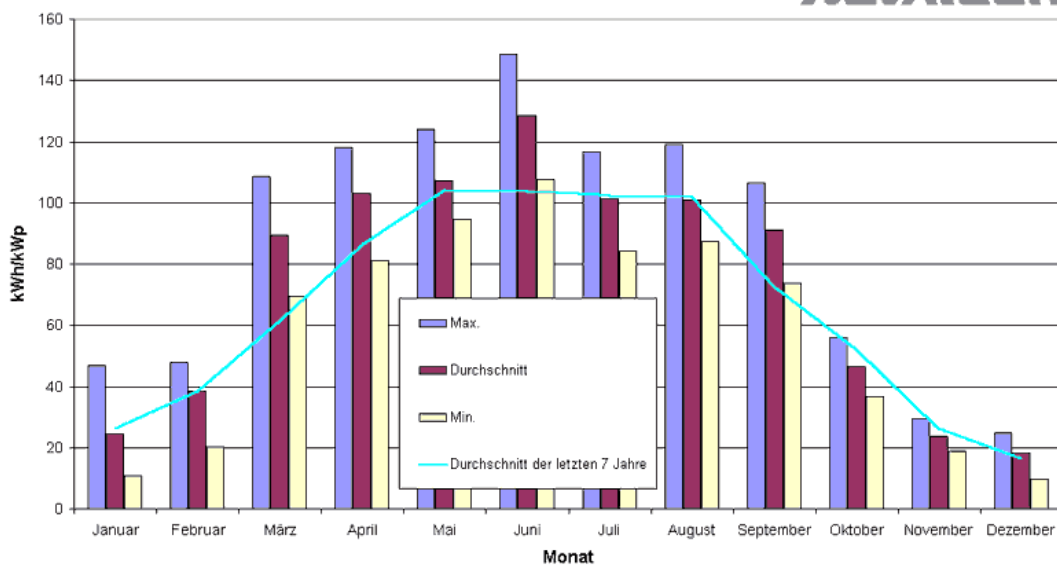
Leistungsstatistik der Fotovoltaikanlagen im Jahr 2002
