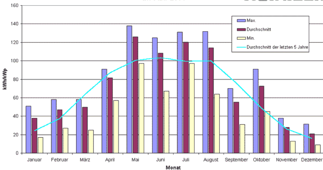
Leistungsstatistik der Fotovoltaikanlagen im Jahr 2001
